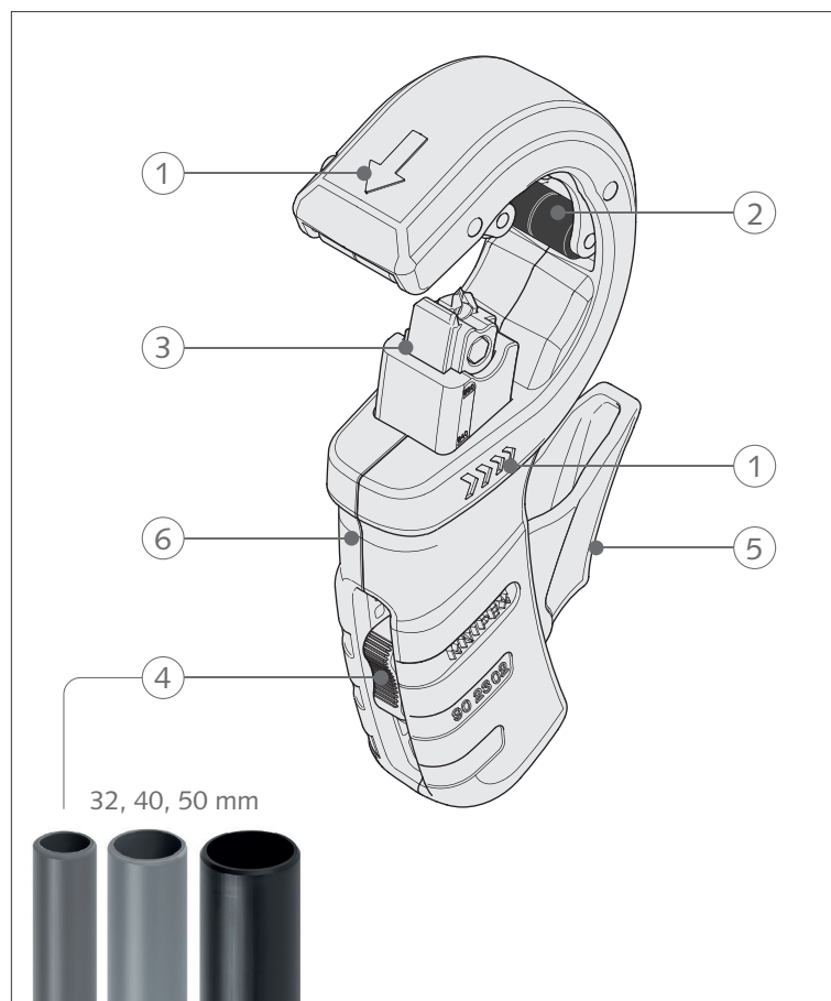
Настройка трубореза DPT50
