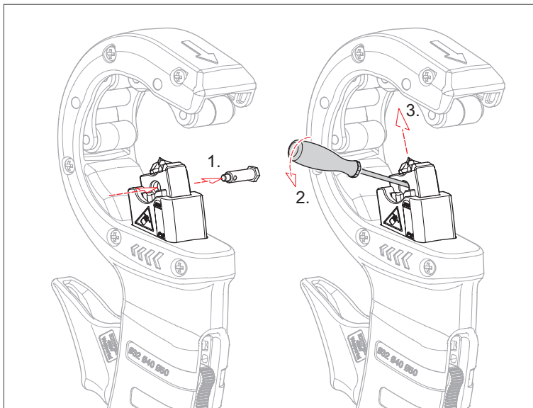
Извлечение лезвия
