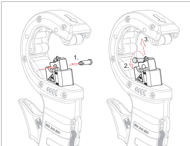
Снятие лезвия
