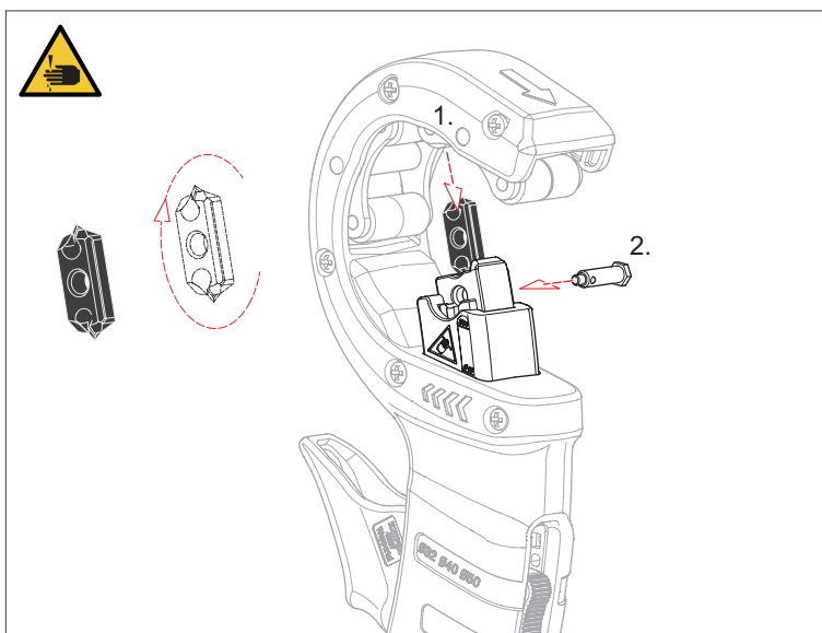
Вставка лезвия
